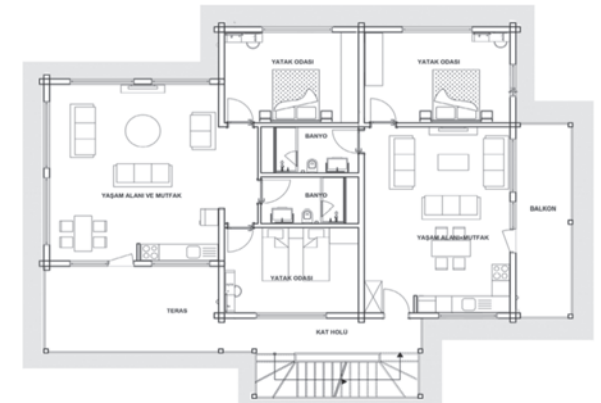
KAT PLANI
