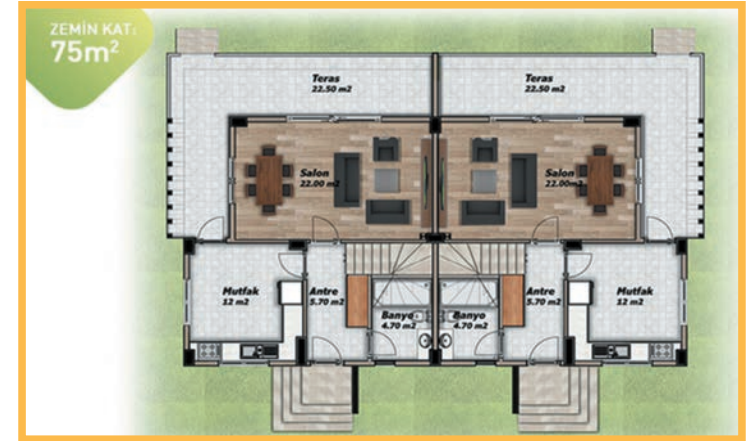
KAT PLANI
