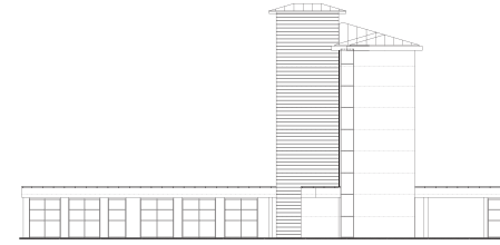
SAĞ YAN CEPHE
