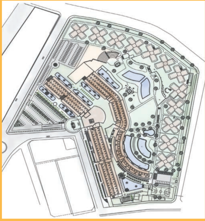
VAZİYET PLANI
